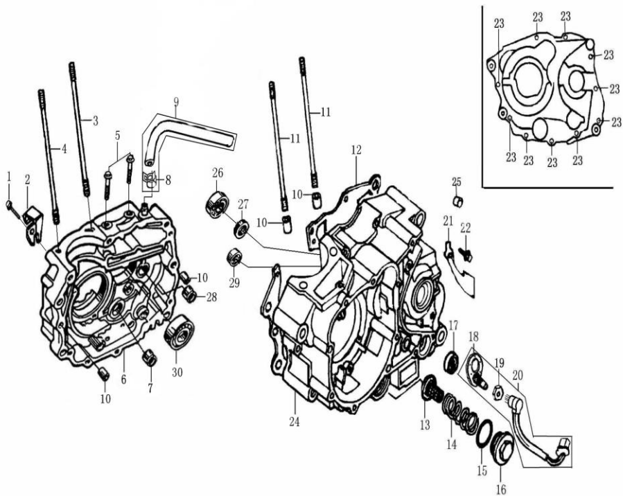
曲轴箱 CRANKCASE
